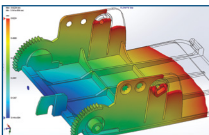
Füllzeit und Schmelzfrontposition einer Füllanalyse in SOLIDWORKS Plastics
