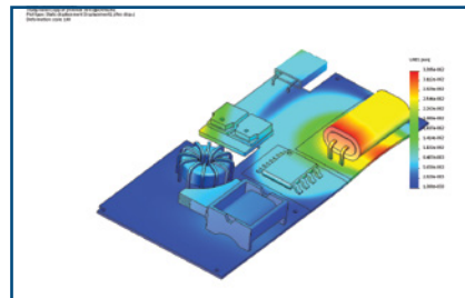
Verschiebungsverteilung einer verknüpften thermischen Spannungsanalyse in SOLIDWORKS Simulation
