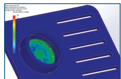
Spannungsverteilung eines Kunststoffteils, das einer externen Belastung gepaart mit Gussform-Restspannungen unterliegt
