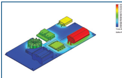
Temperaturverteilung einer CFD-Analyse in SOLIDWORKS Flow Simulation
