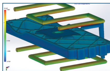
Wärmefluss einer SOLIDWORKS Plastics Kühlsimulation des Hohlraums, der Kühlkanäle und der Gussform
