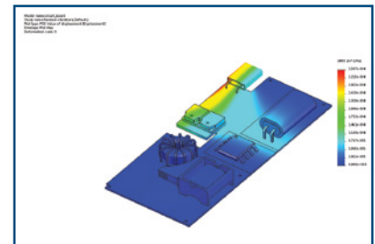
Spektrale Leistungsdichte (PSD)-Werte aus einer Zufallsvibrationsanalyse in SOLIDWORKS Simulation
